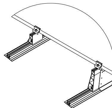
Mostek H30 L=330 / Bridge H30 L=330
